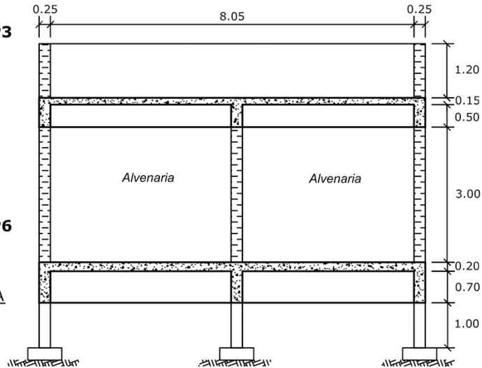
Corte AA
